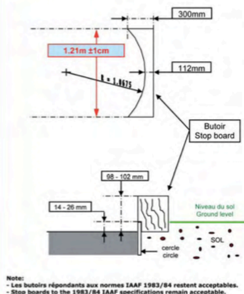
DIAMETRE INTERIEUR DU CERCLE / INSIDE DIAMETER = 2m135 (+ ou - 5mm)
